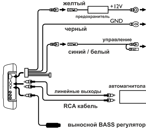
A. Схема подключения сабвуфера к головному устройству через НЧ линейные входы RCA
