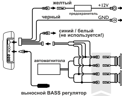
B. Схема подключения сабвуфера к головному устройству по высокоуровневым входам (к динамикам)
